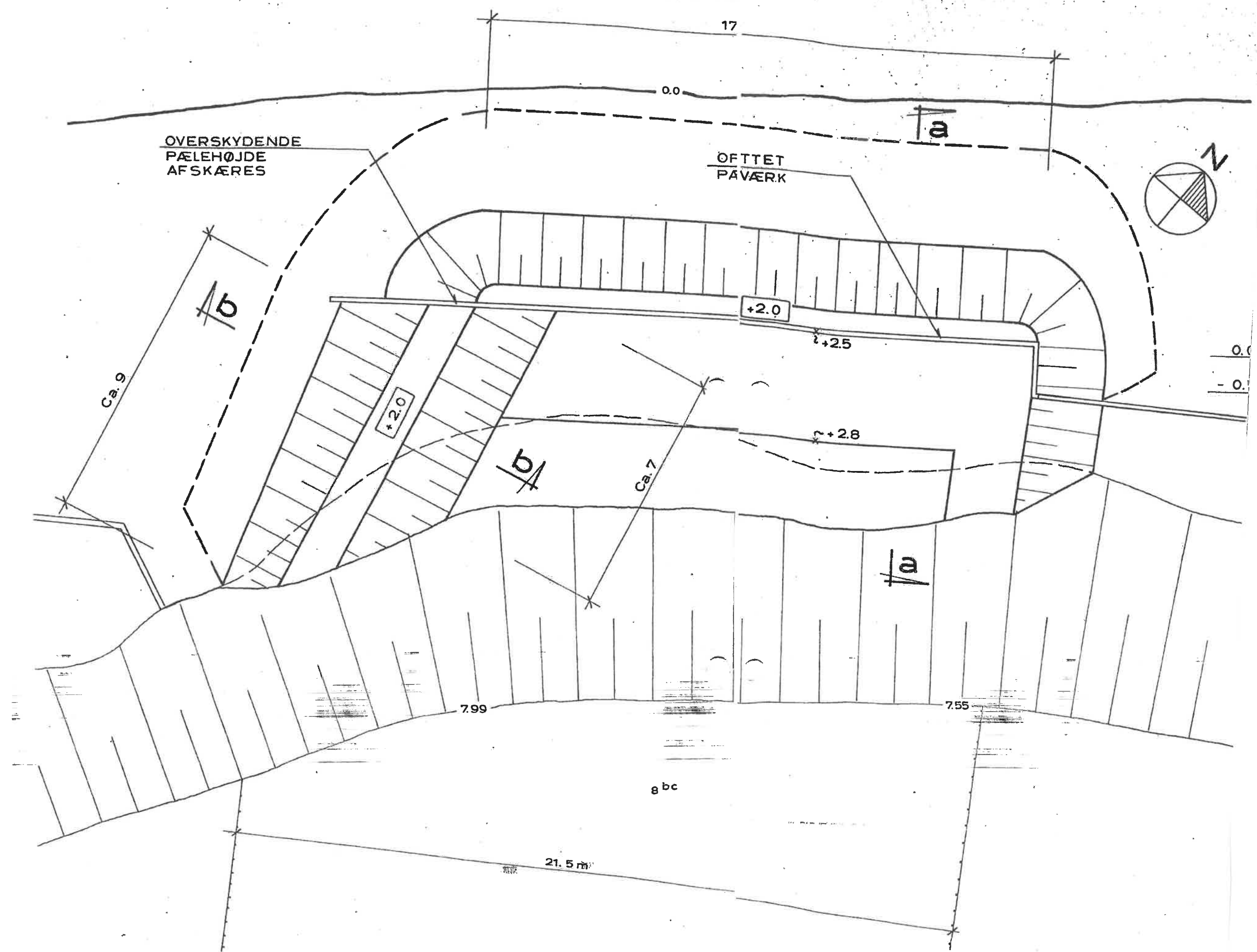
PLAN, 1:100
